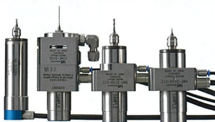
電動モータスピンドルシリーズ E3000i
